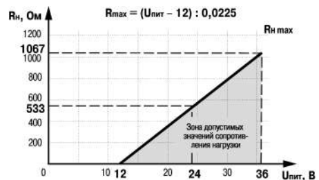
Рисунок 2.1 – График для выбора допустимых значений сопротивления нагрузки
